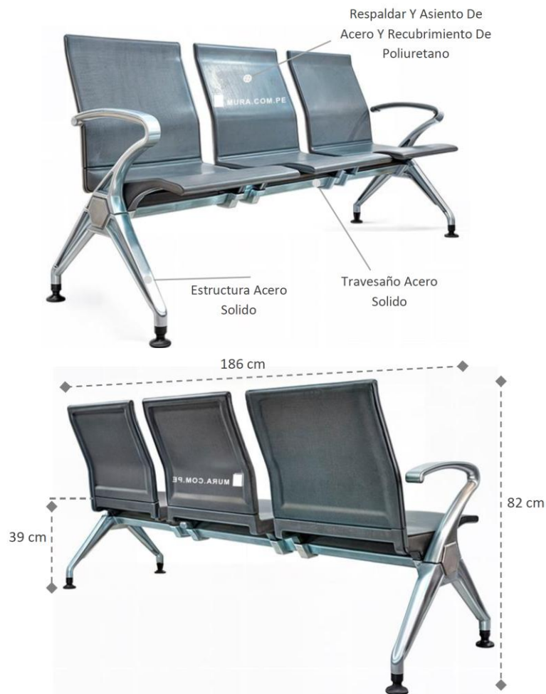
Imágenes referenciales de banca de asientos múltiples de metal - 3 asientos
